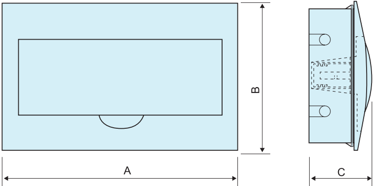
Planos de dimensiones de caja para montaje superficial
