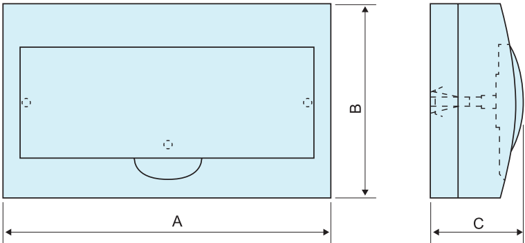
Planos de dimensiones de caja para montaje superficial
