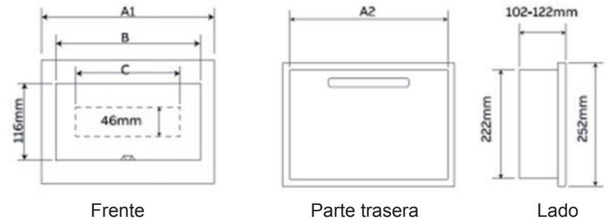
Planos dimensionales de caja de distribución montada en superficie
