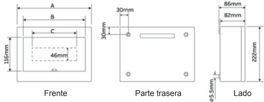
Planos dimensionales de caja de distribución montada en superficie
